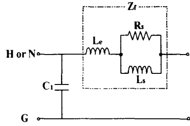
(a) 차동모드(Differential-Mode)
