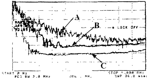
(b) IEC 61000-4-4의 level 3
