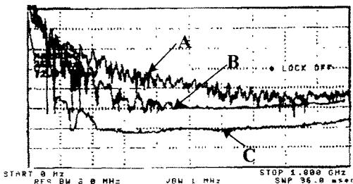
(c) IEC 61000-4-4의 level 4
