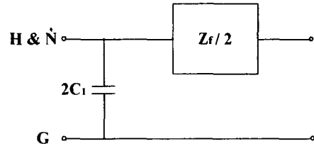
(b) 공통모드(Common-Mode)
