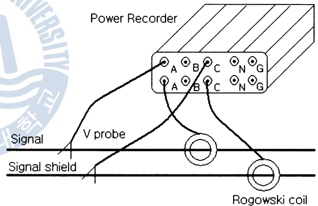
(a) 결선도
