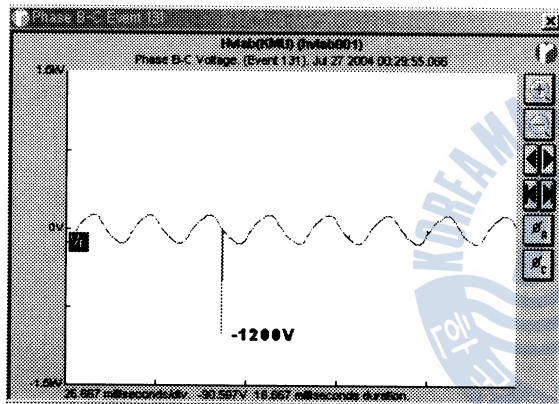
(a) 서지 파형 1
