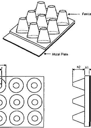
그림 2. 꼭지절단 원추형 전파흡수체
