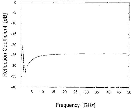
그림 5. 꼭지절단 원추형 전파흡수체의 주파수특성
