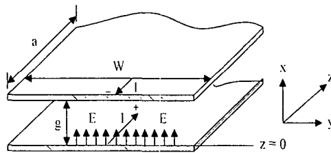
그림 1. 평행판 전송선로
