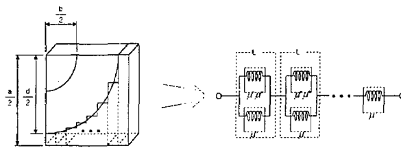
그림 4. 2층부의 등가투자율 모델
