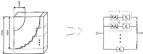
그림 3. 2층부의 등가유전을 모델
