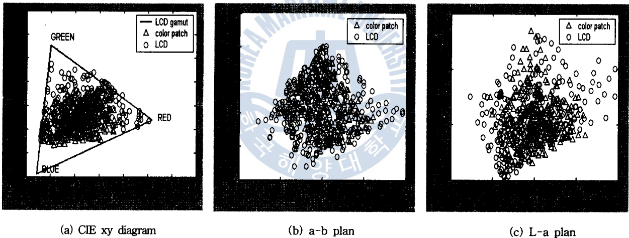
(그림 5) 보정전 색표와 LCD 모니터의 측정치 분포
